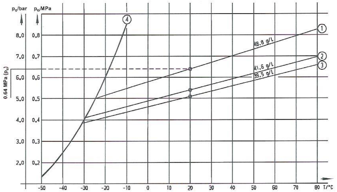
Curva de pressão de SF 6 -30°C (ND = 0,64 MPa ( p_e ) / UW1 = 0,54 MPa ( p_e ) / UW2 = 0,51 MPa ( p_e ))
